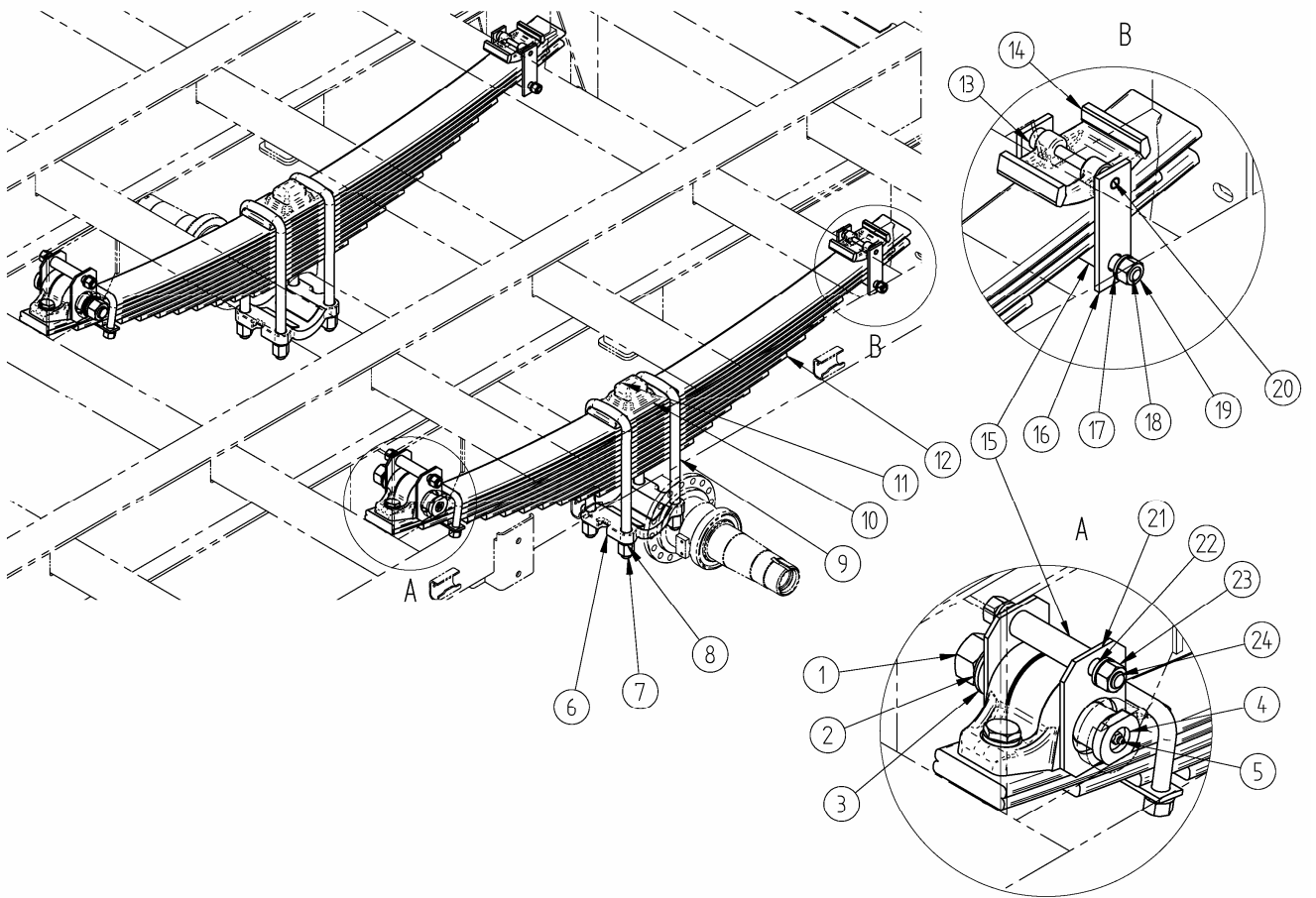
Рисунок 13 – Задняя подвеска 8543-01, 85431-01 Примечание: 1, 2, 3, 8, 11, 15 см. в подгруппе 2902
