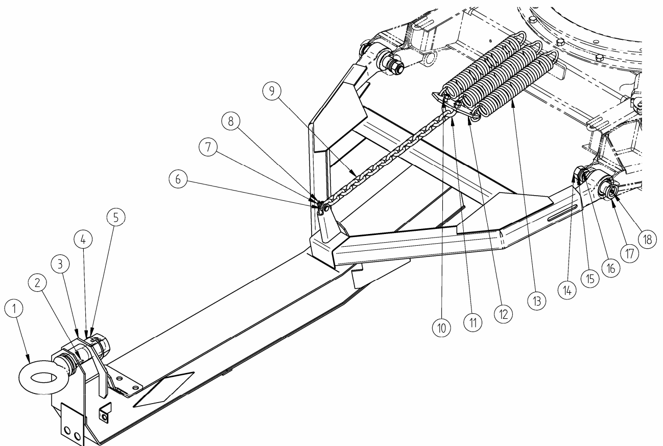
Рисунок 8 – Дышло 8543, 8543-01 Примечание: поз. 14, 15, 16 см. в подгруппе 2902; поз. 17 см. в подгруппе 2902 (для п. 8543) и 2912 (для п. 8543-01)
