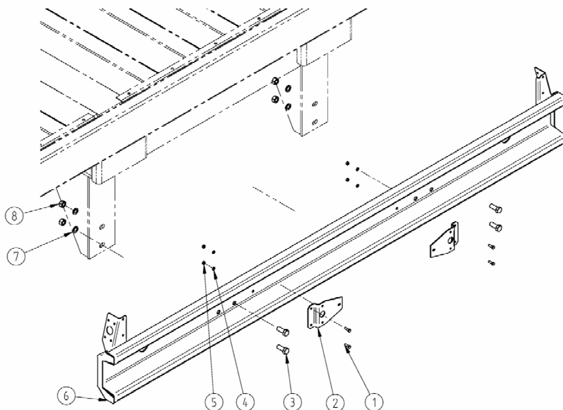
Рисунок 11 – Бампер
