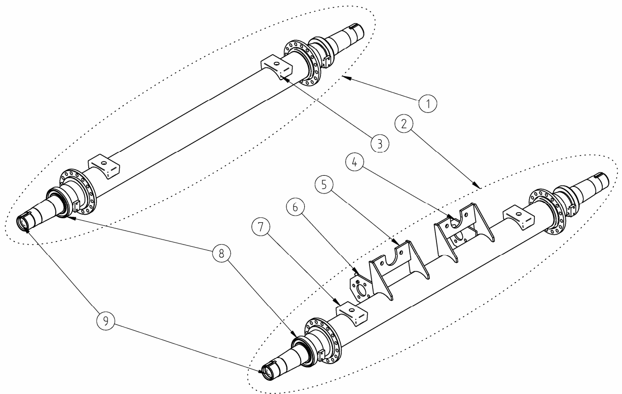
Рисунок 4 – Балки осей
