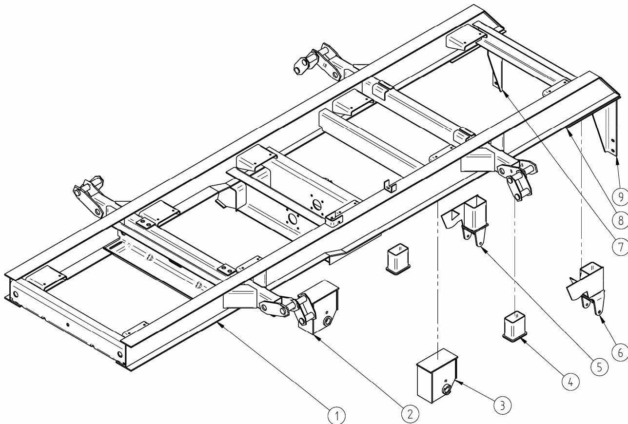
Рисунок 9 – Рама прицепа 8543-01, 85431-01
