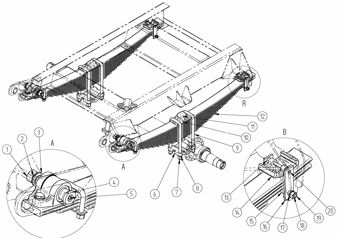
Рисунок 14 – Передняя подвеска 8543-01, 85431-01 Примечание: 1, 2, 3, 8, 11, 15 см. в подгруппе 2902
