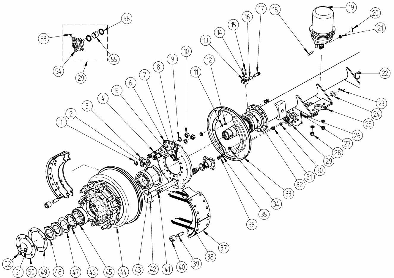
Рисунок 2 – Ось 8543-01, 85431-01 (длинный кулак)
