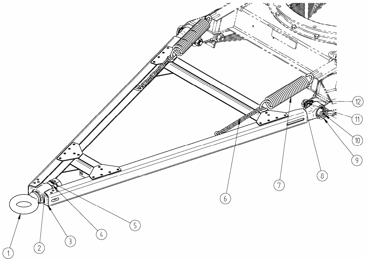
Рисунок 7 – Дышло 85431, 85431-01 Примечание: поз. 8, 11, 12 см. в подгруппе 2902; поз. 9 см. в подгруппе 2902 (для п. 85431) и 2912 (для п. 85431-01)
