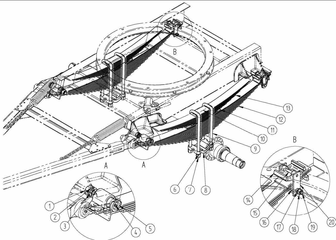
Рисунок 12 – Подвеска 8543, 85431
