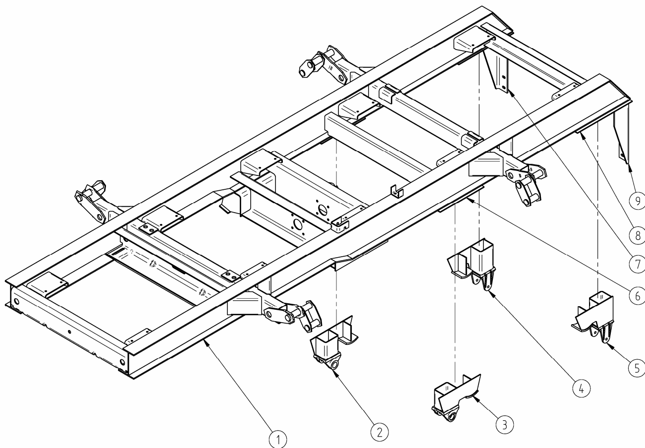
Рисунок 10 – Рама прицепа 8543, 85431
