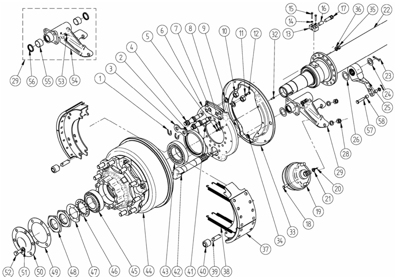
Рисунок 3 – Ось 8543, 85431 (короткий кулак)
